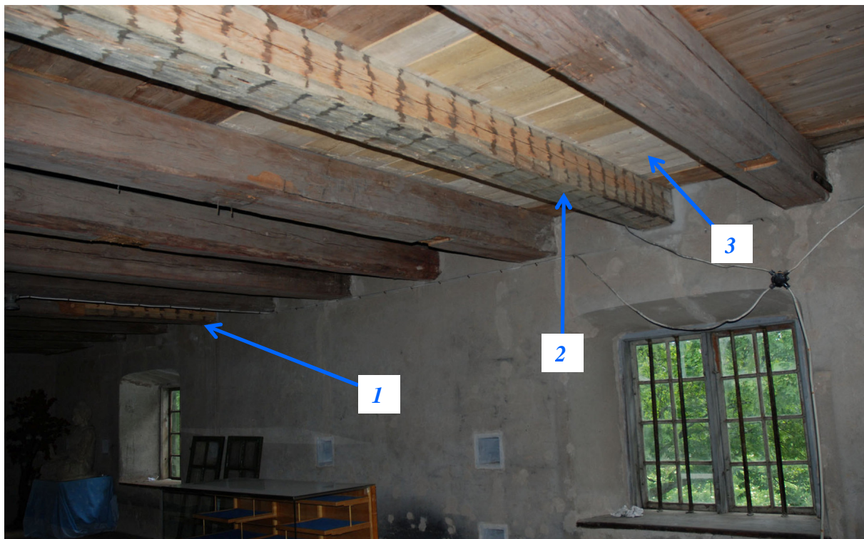
Nummer 1 markerar var rötskadad bjälke lagats. 2 markerar ny del av bjälke som monterats där bjälke tidigare var avsågad. 3 markerar nytt golvvirke.
