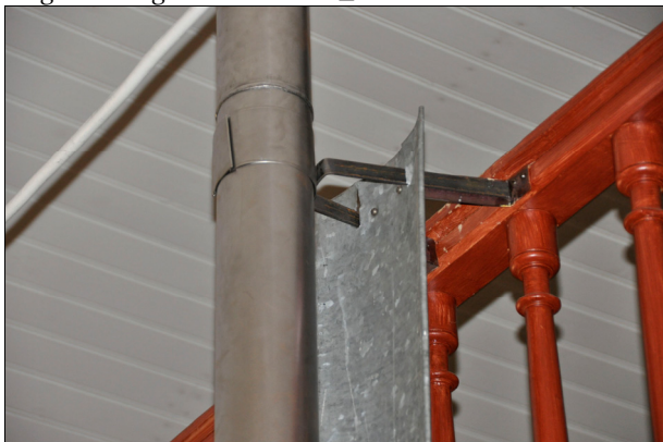
Den nya övre hållaren på rökröret har monterats fram till rökröret för att begränsa dess rörlighet. Bildnr Vlm_kmvIM-2640.
