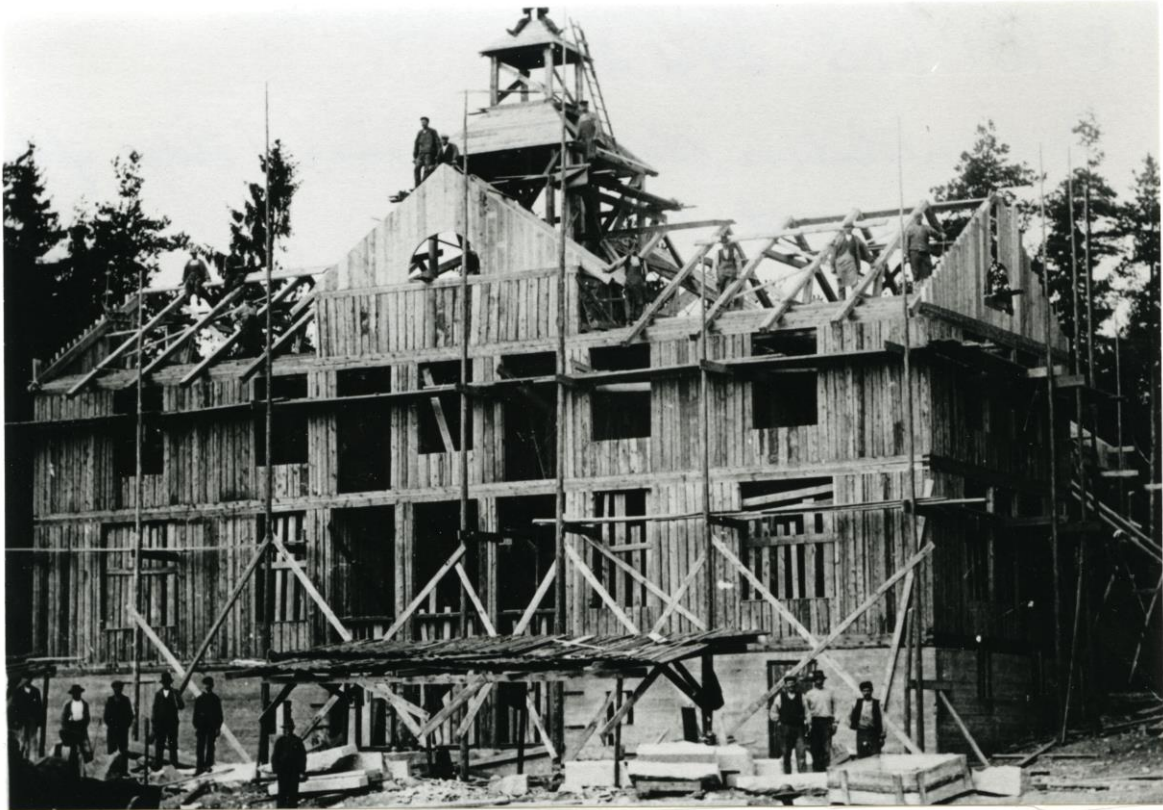
Bultlokalen under uppförande 1913. Stomme av stående timmer. Fotograf okänd. Västmanlands läns museums arkiv, bildid Vlm-B 101 605-25.
